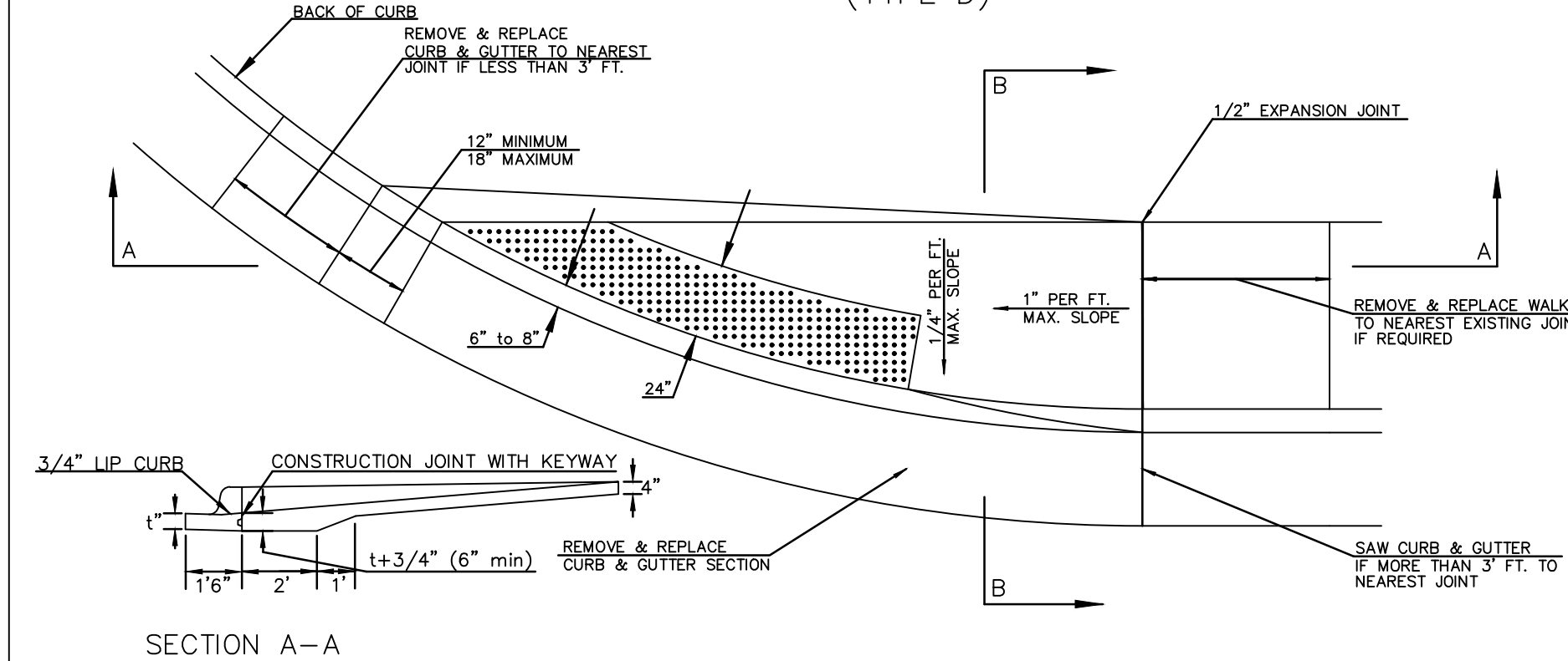
SECTION A-A
