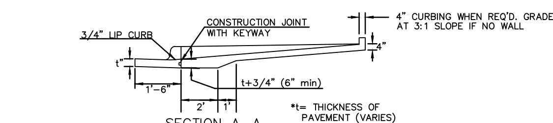
SECTION A-A
