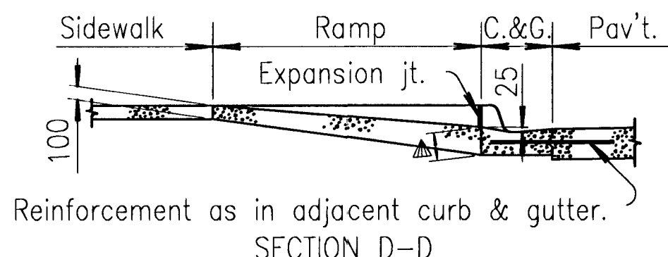
SECTION D-D
