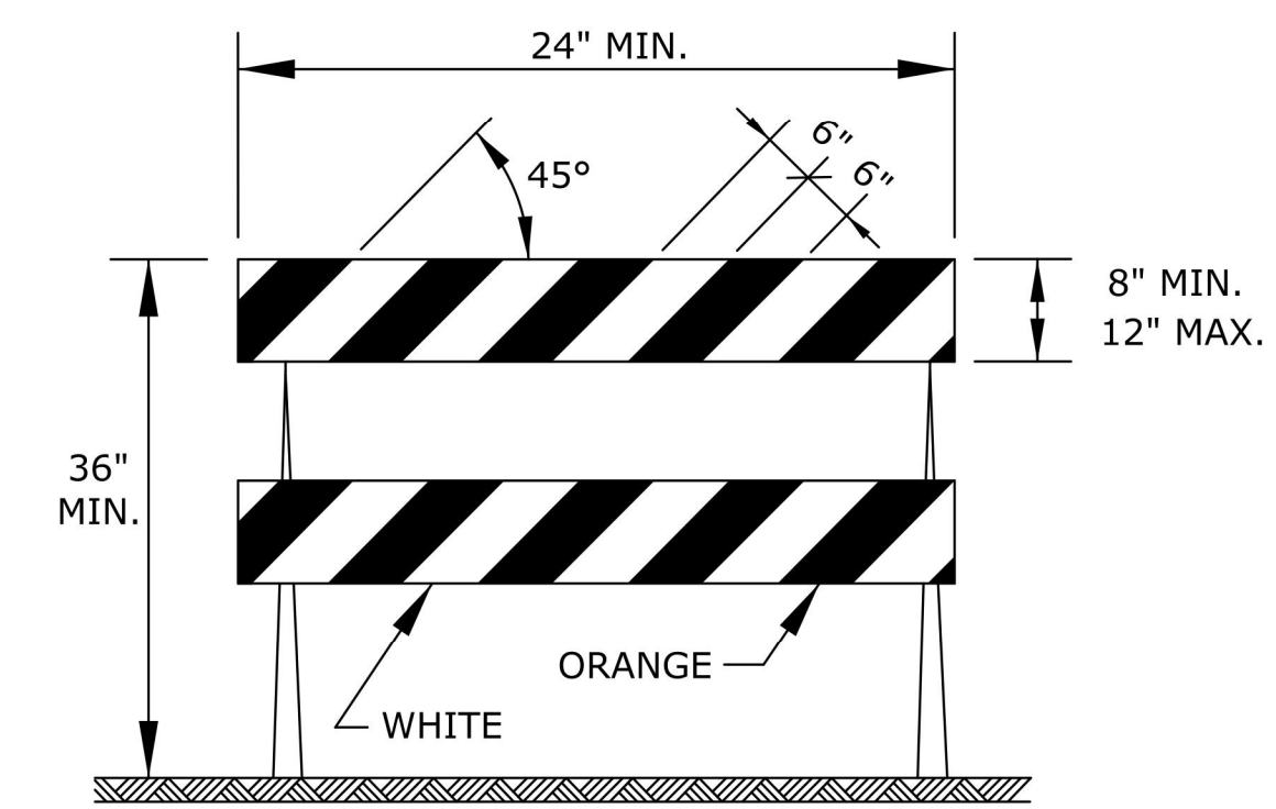
TYPE 2 BARRICADE
