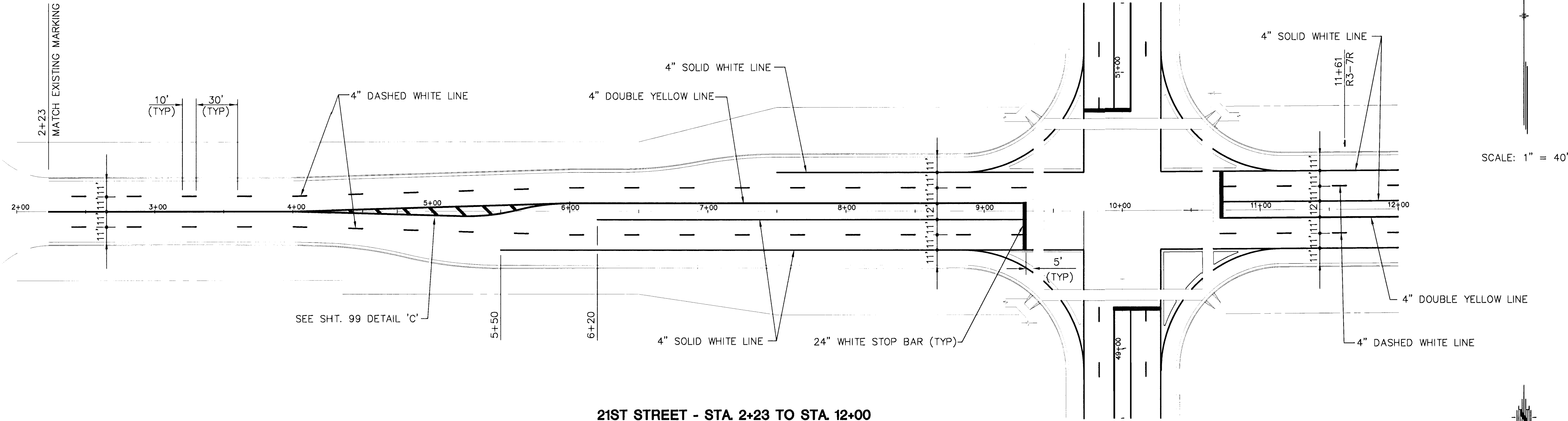
21ST STREET - STA. 2+23 TO STA. 12+00
