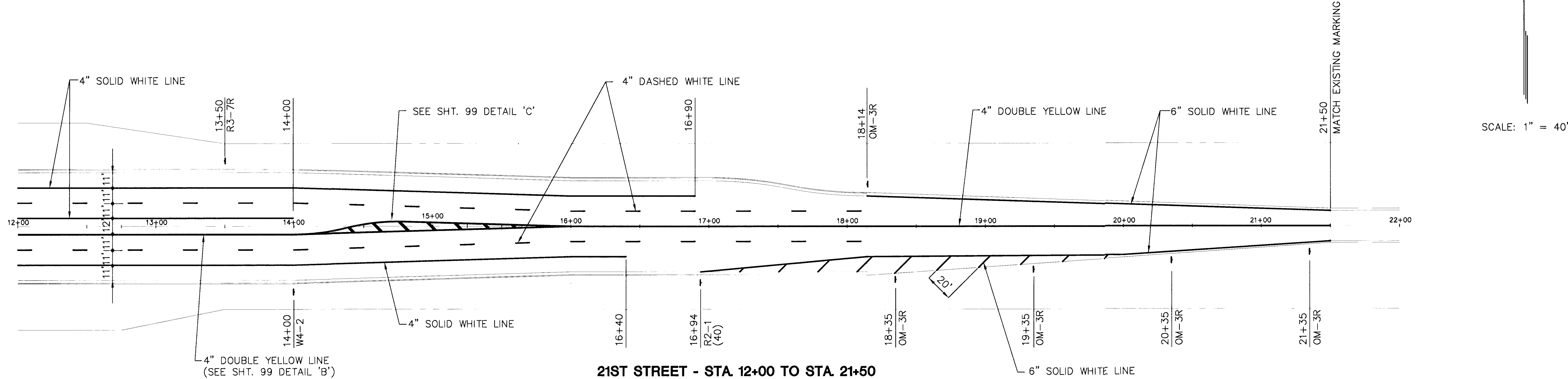
21ST STREET - STA. 12+00 TO STA. 21+50
