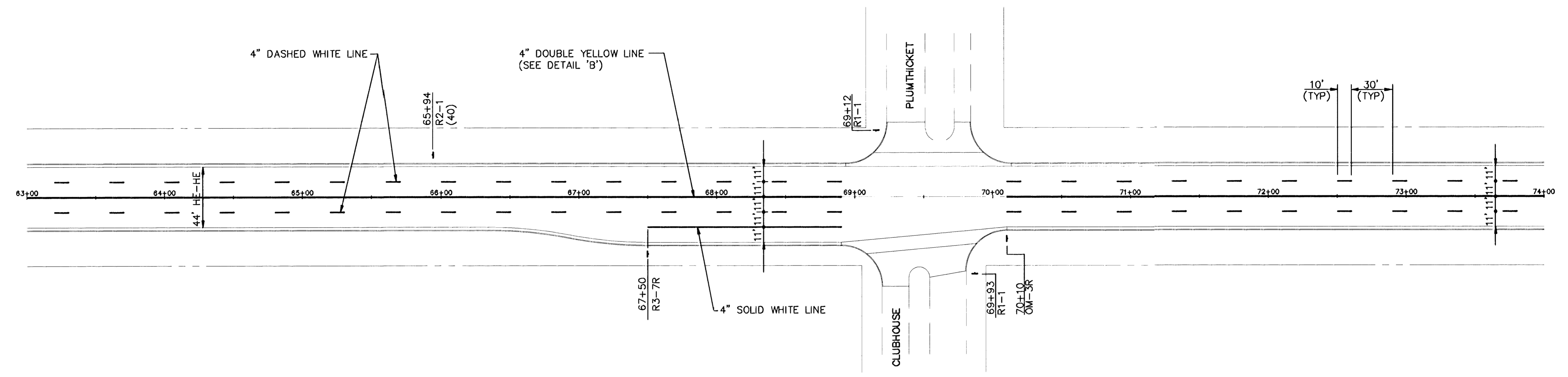
WEBB ROAD - STA. 63+00 TO STA. 74+00
