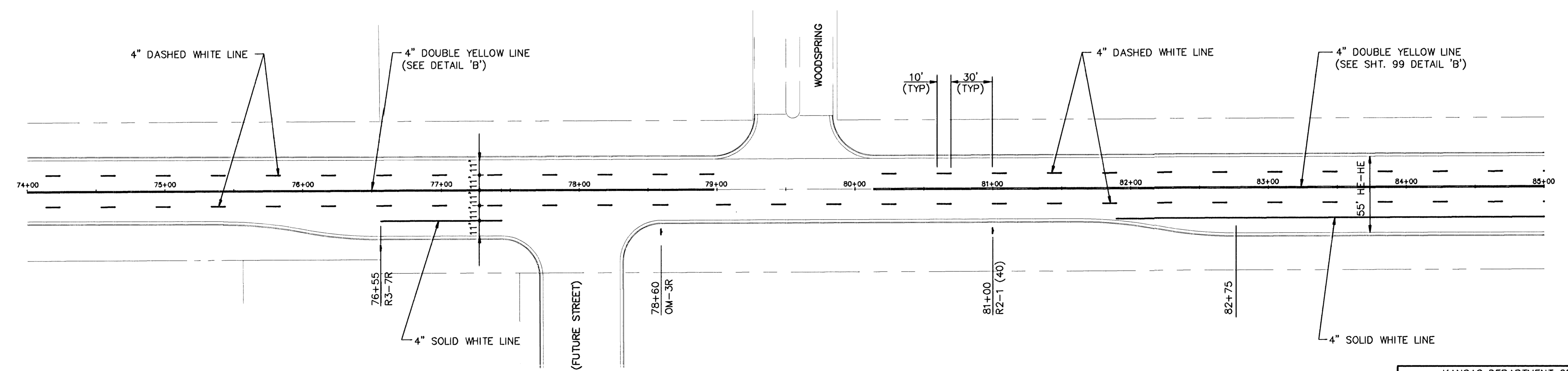
WEBB ROAD - STA. 74+00 TO STA. 85+00
