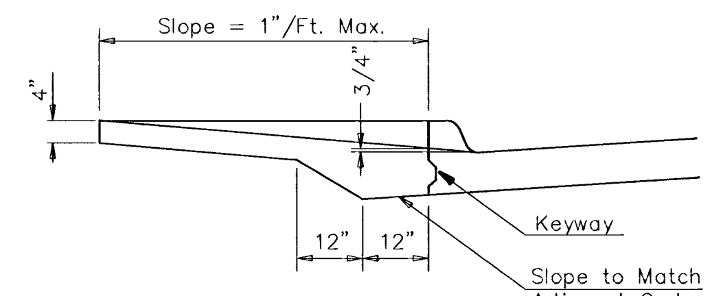
SECTION A-A
