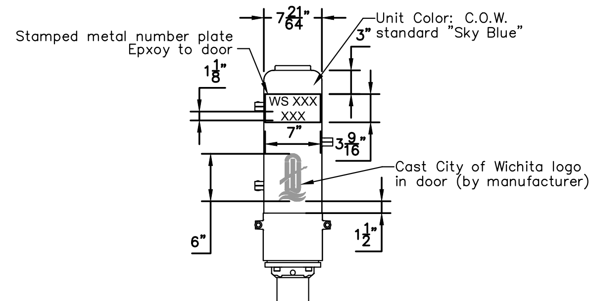
Door Detail
