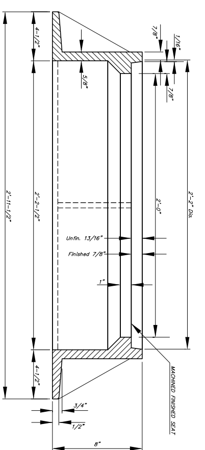
SECTION A-A
