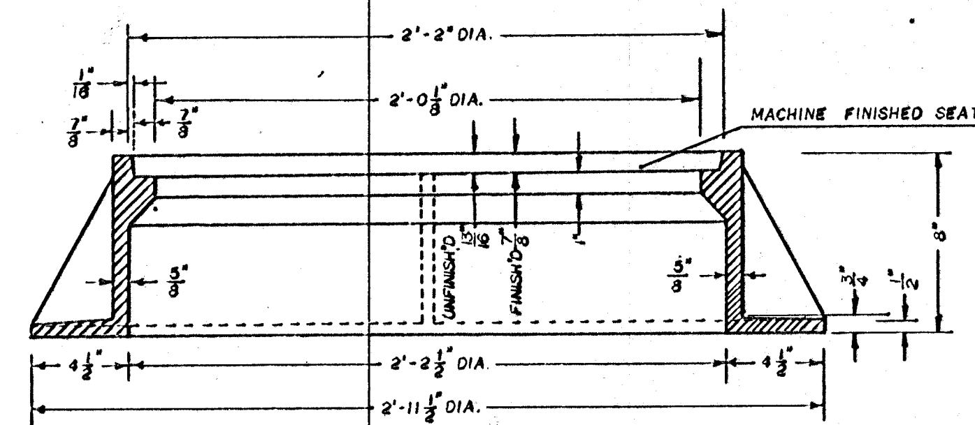
SECTION A-A
