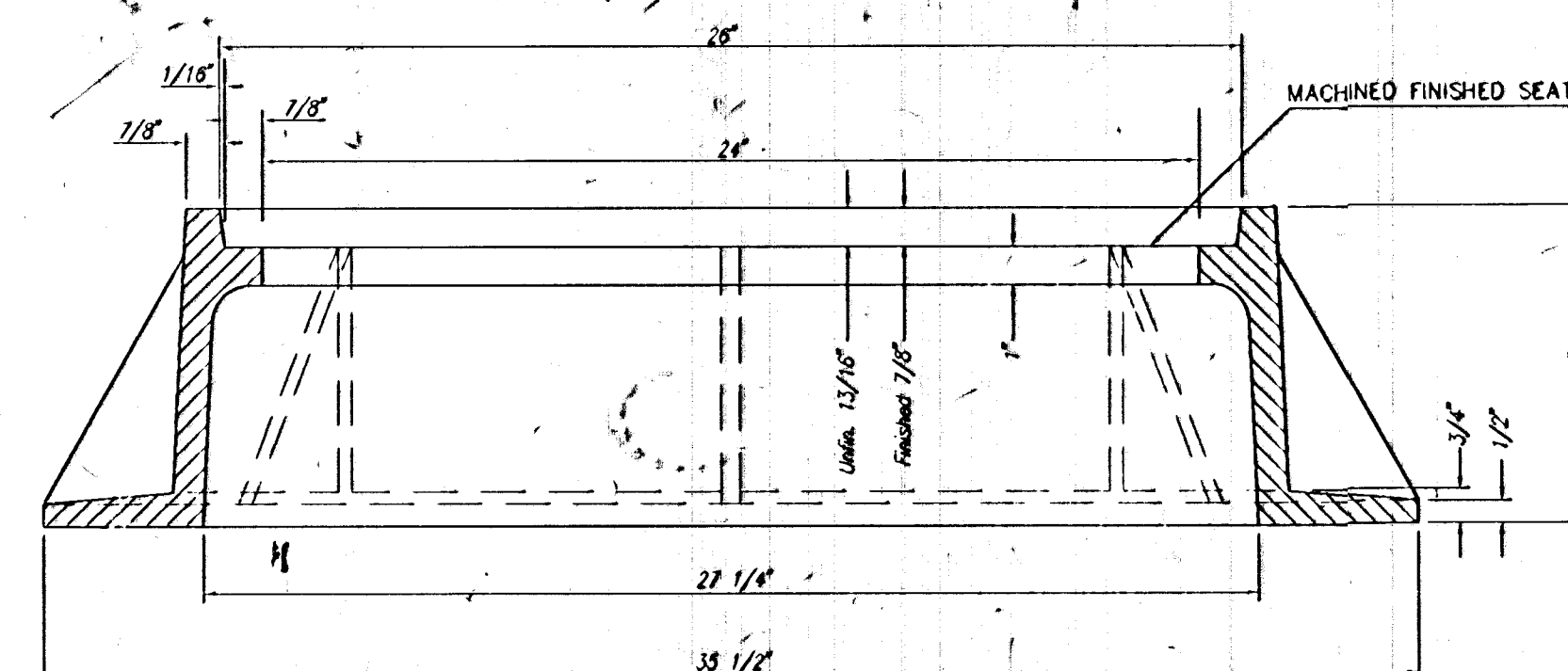
SECTION A-A
