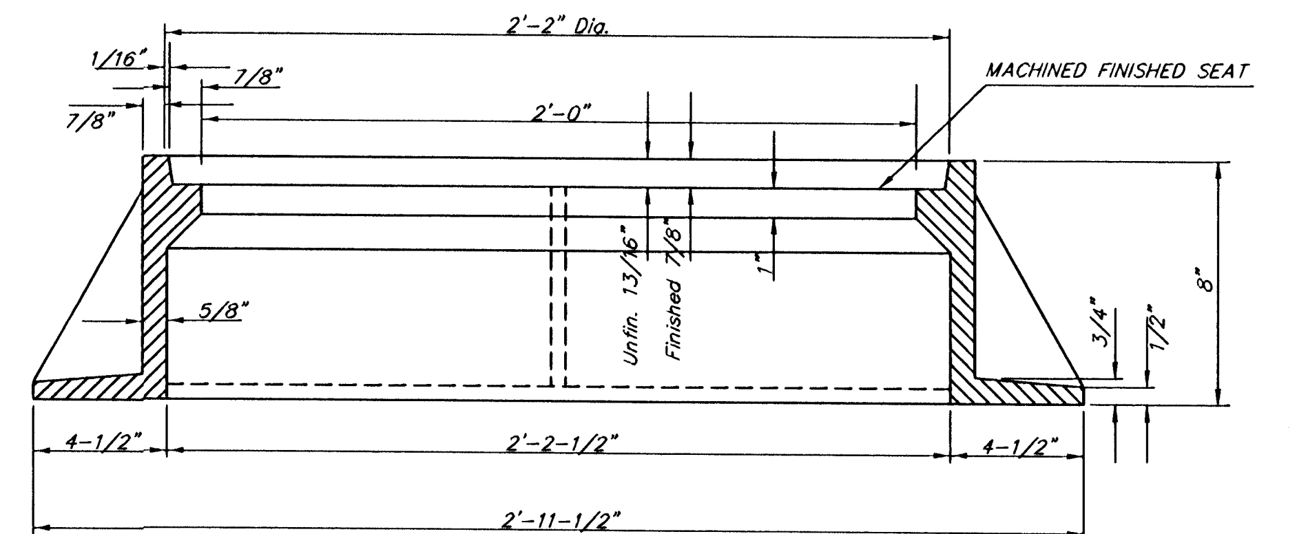
SECTION A-A
