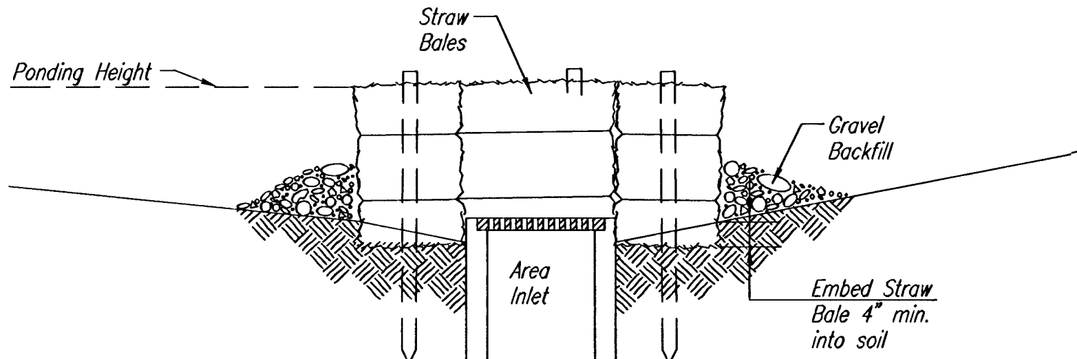
SECTION A-A
