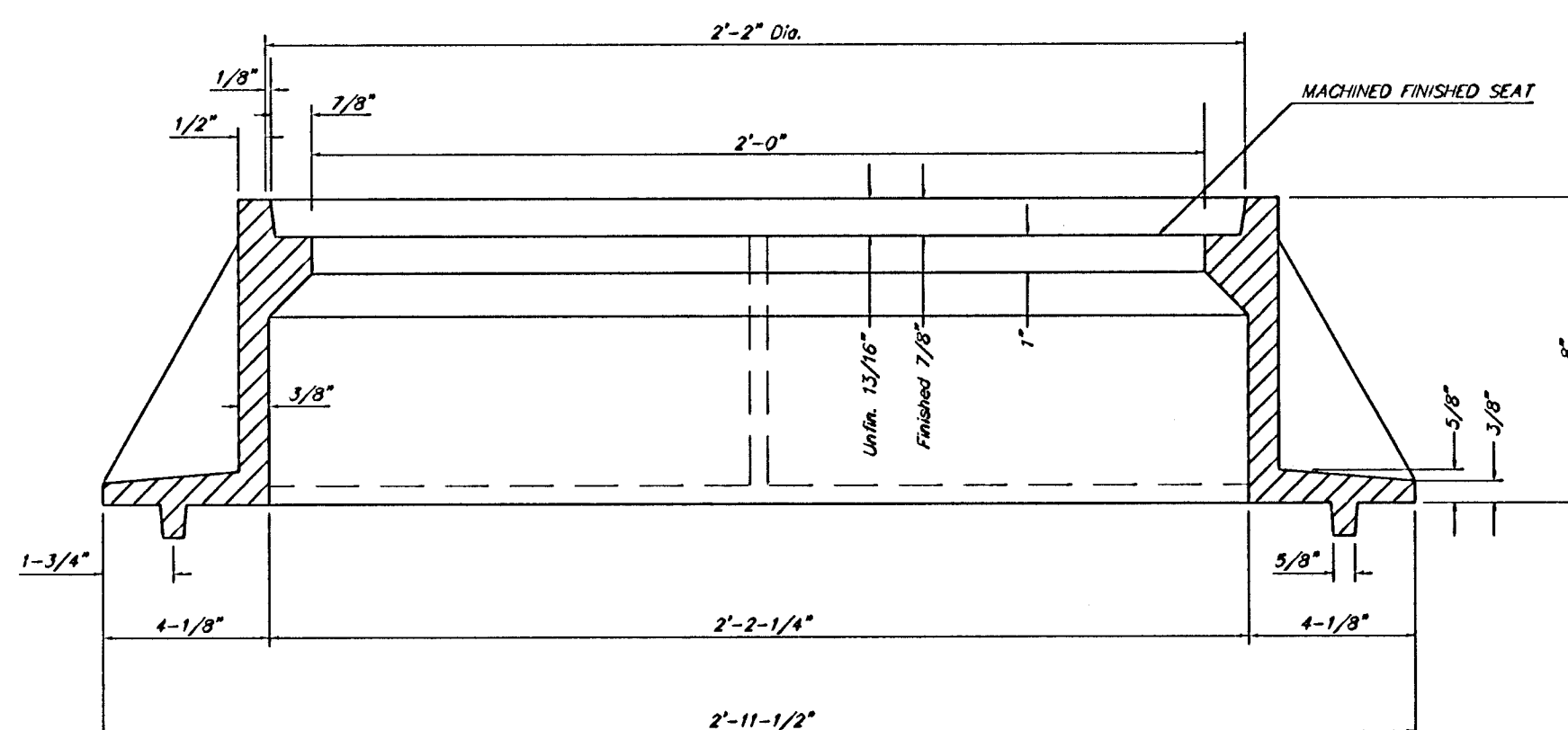
SECTION A-A
