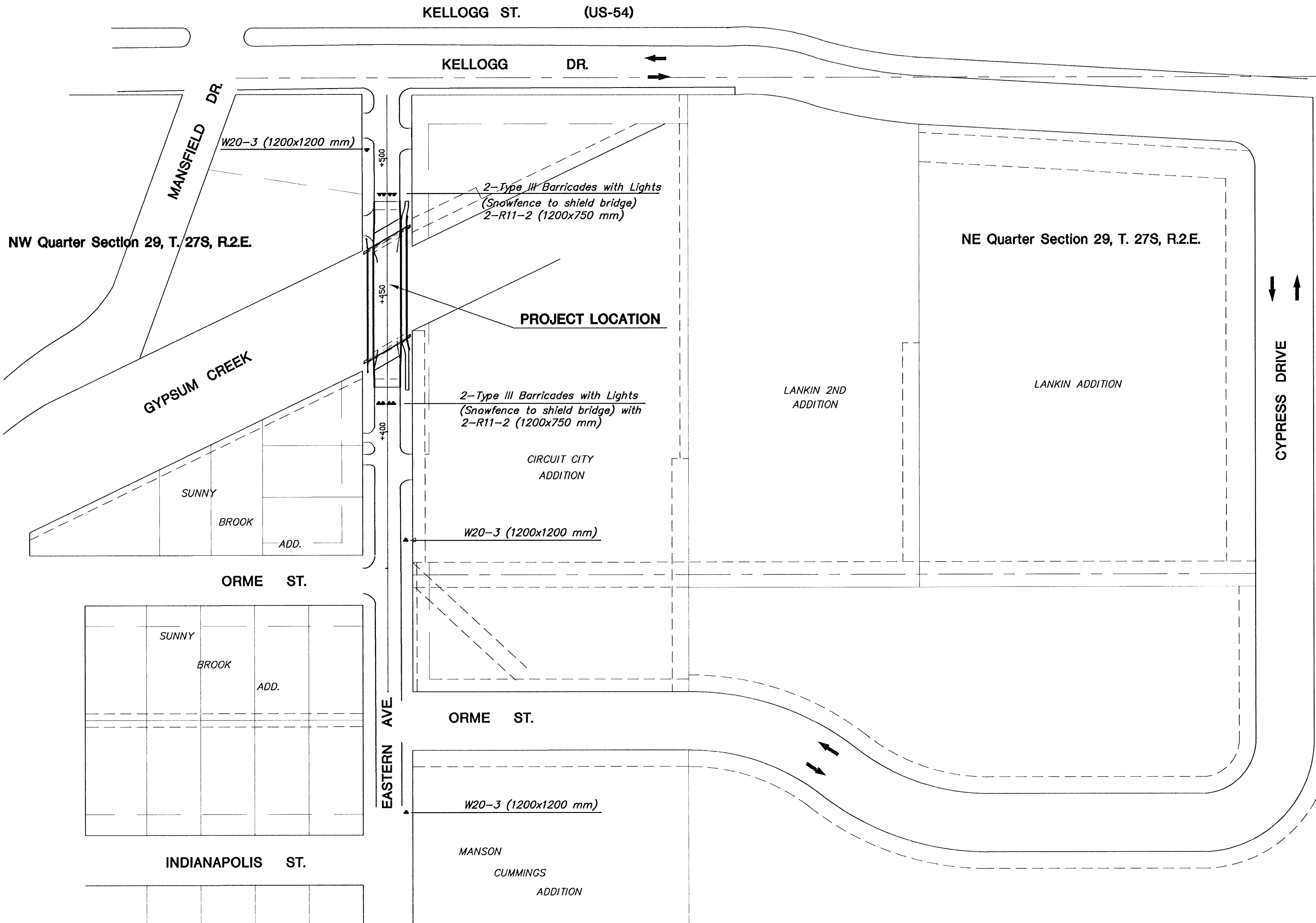
DETOUR PLAN
