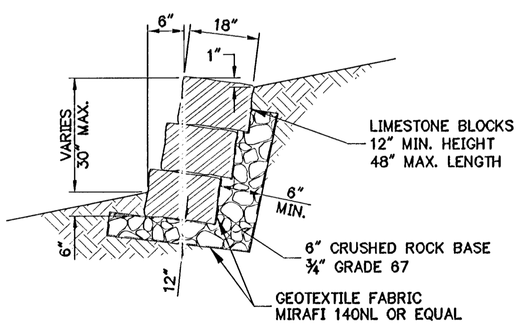
TYPE "B" WALL SCALE: N.T.S.
