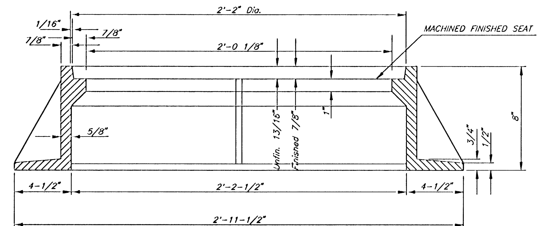
SECTION A-A
