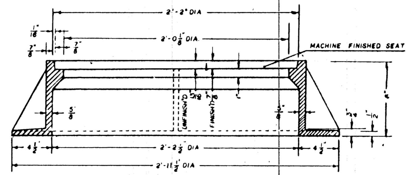
SECTION A-A
