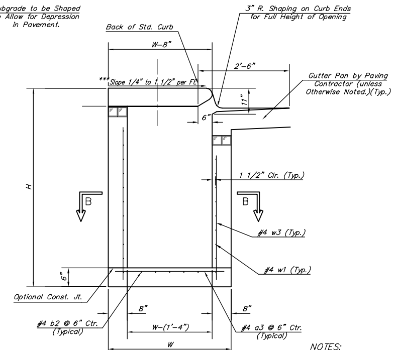
SECTION D-D
