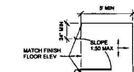
3 TYP STOOP 1/4" = 1'-0"
