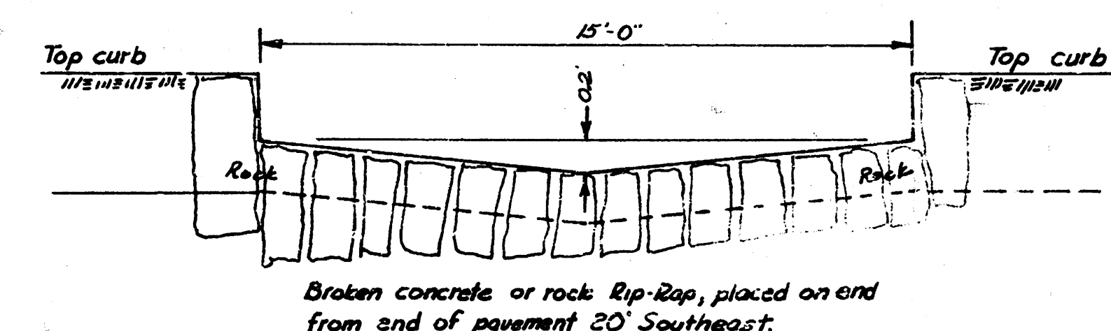
SECTION A-A
