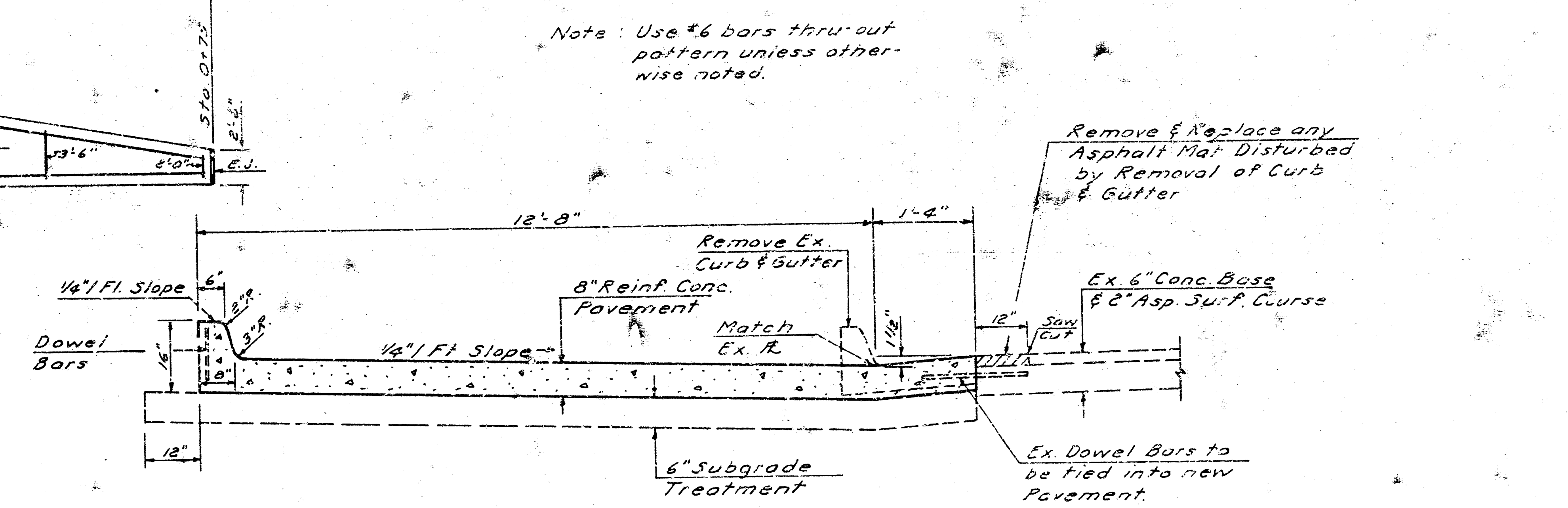
SECTION A-A
