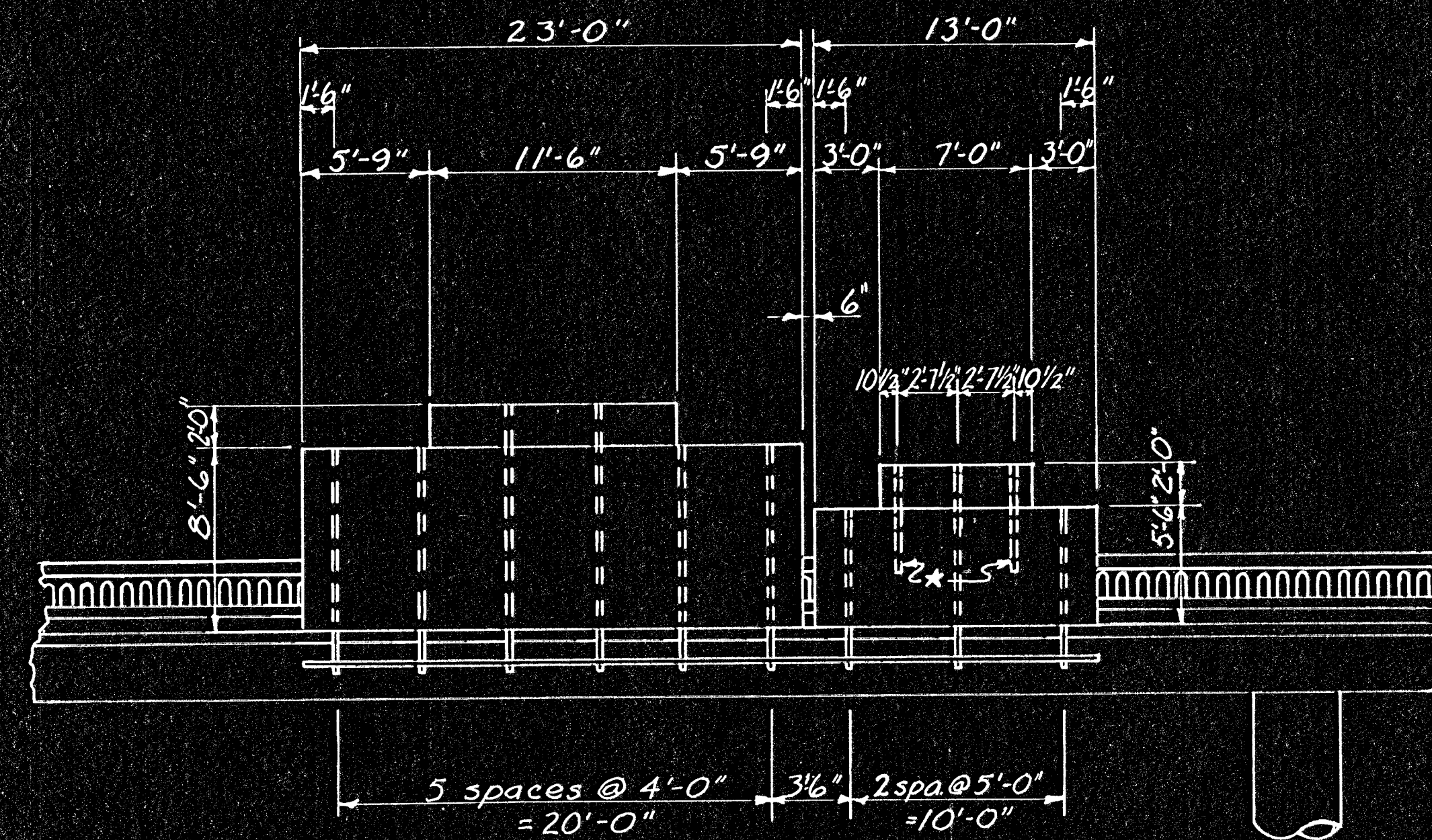
ELEVATION
