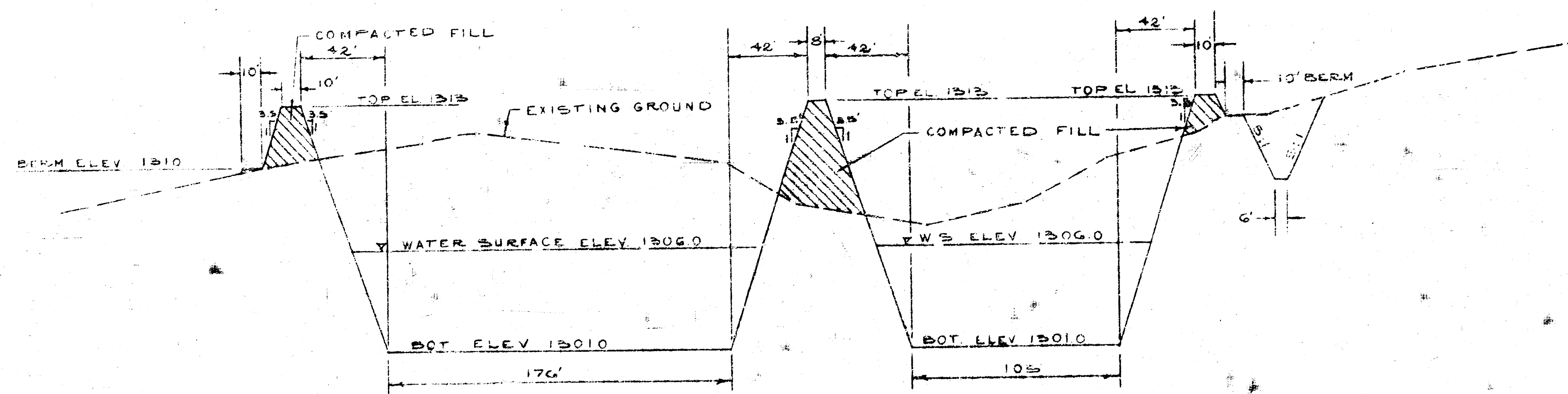
SECTION B-B HORIZ - 1\"/>
