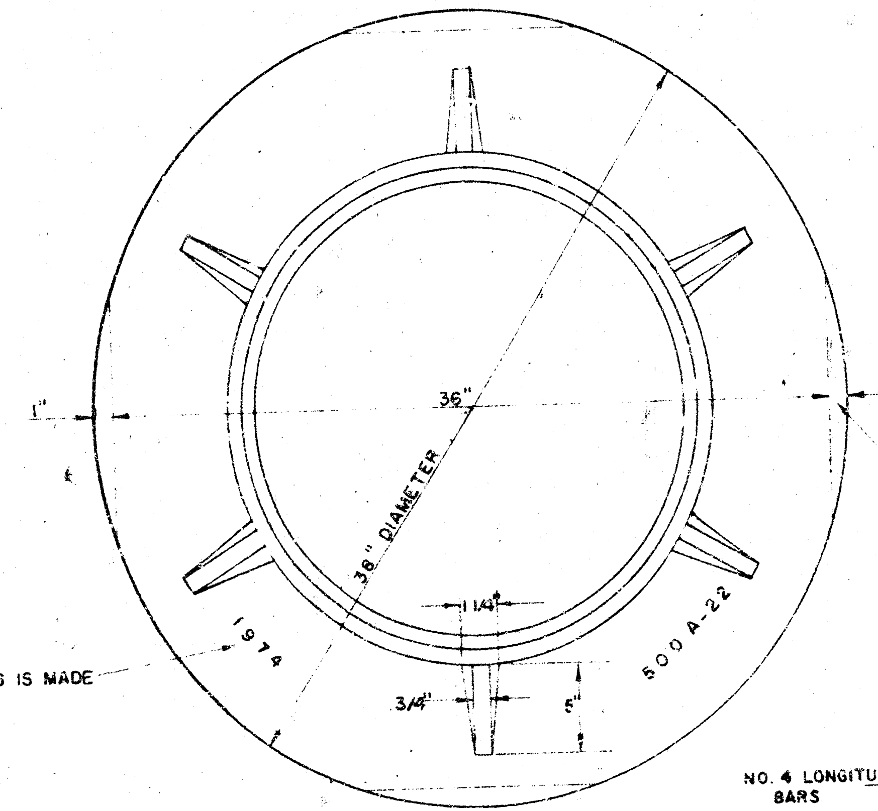
MANHOLE RING
