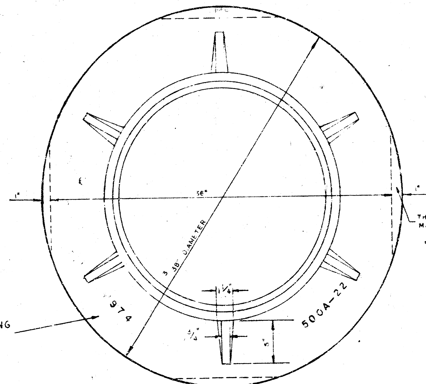
MANHOLE RING
