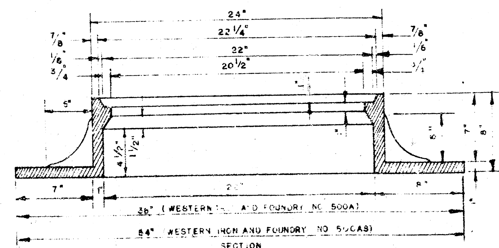
MANHOLE RING
