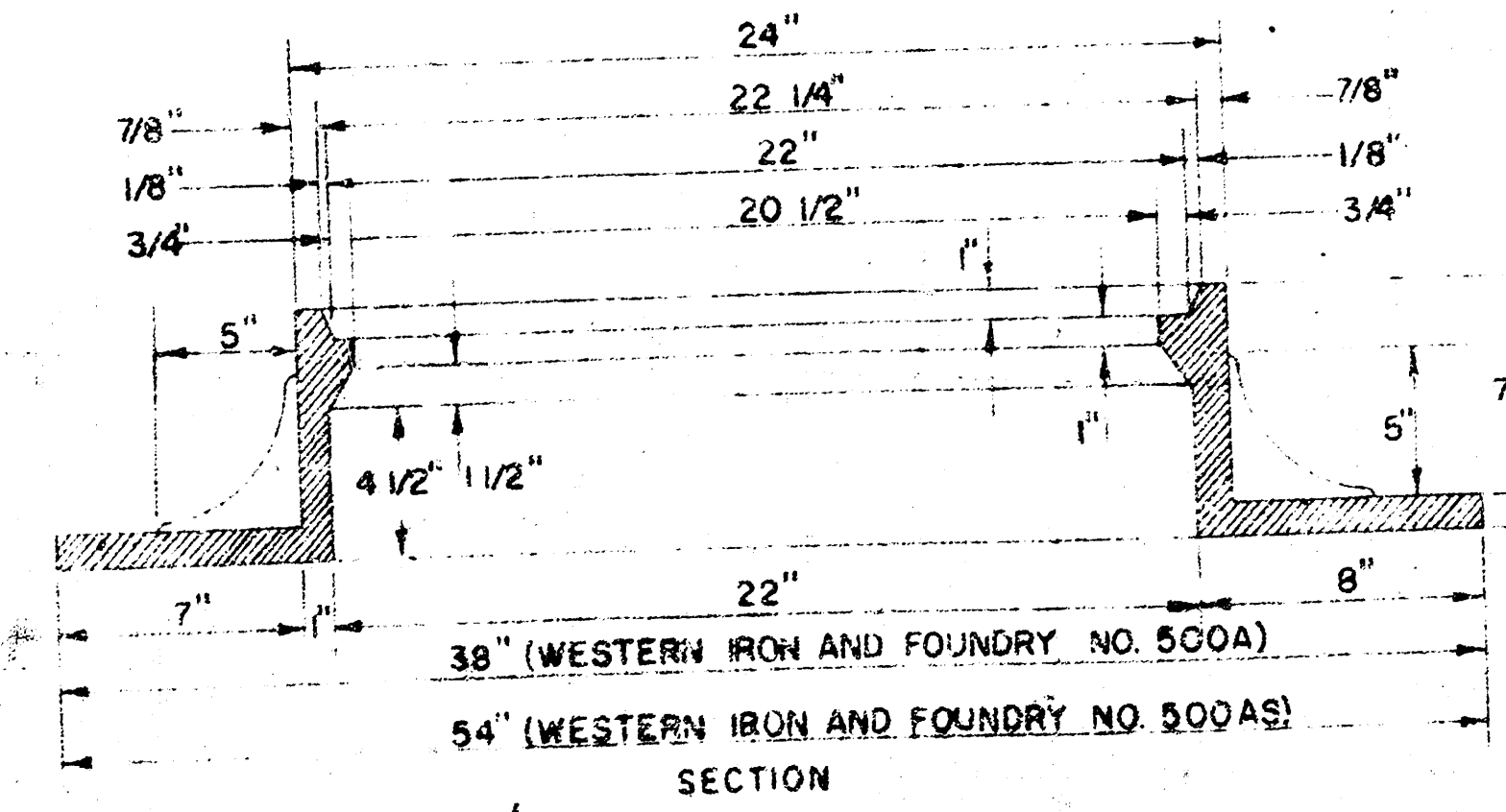
MANHOLE RING
