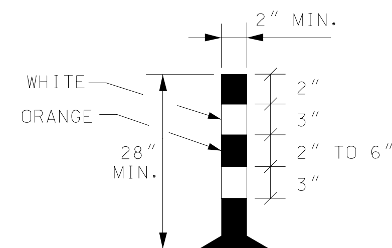
TUBULAR MARKER
