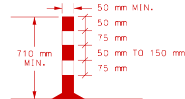
TUBULAR MARKERS
