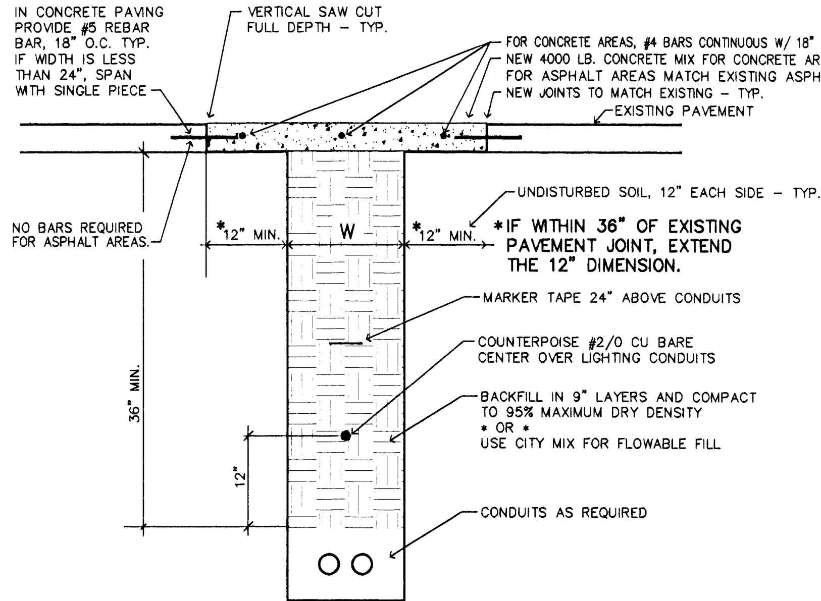
TRENCH BELOW PAVEMENT DETAIL N.T.S.
