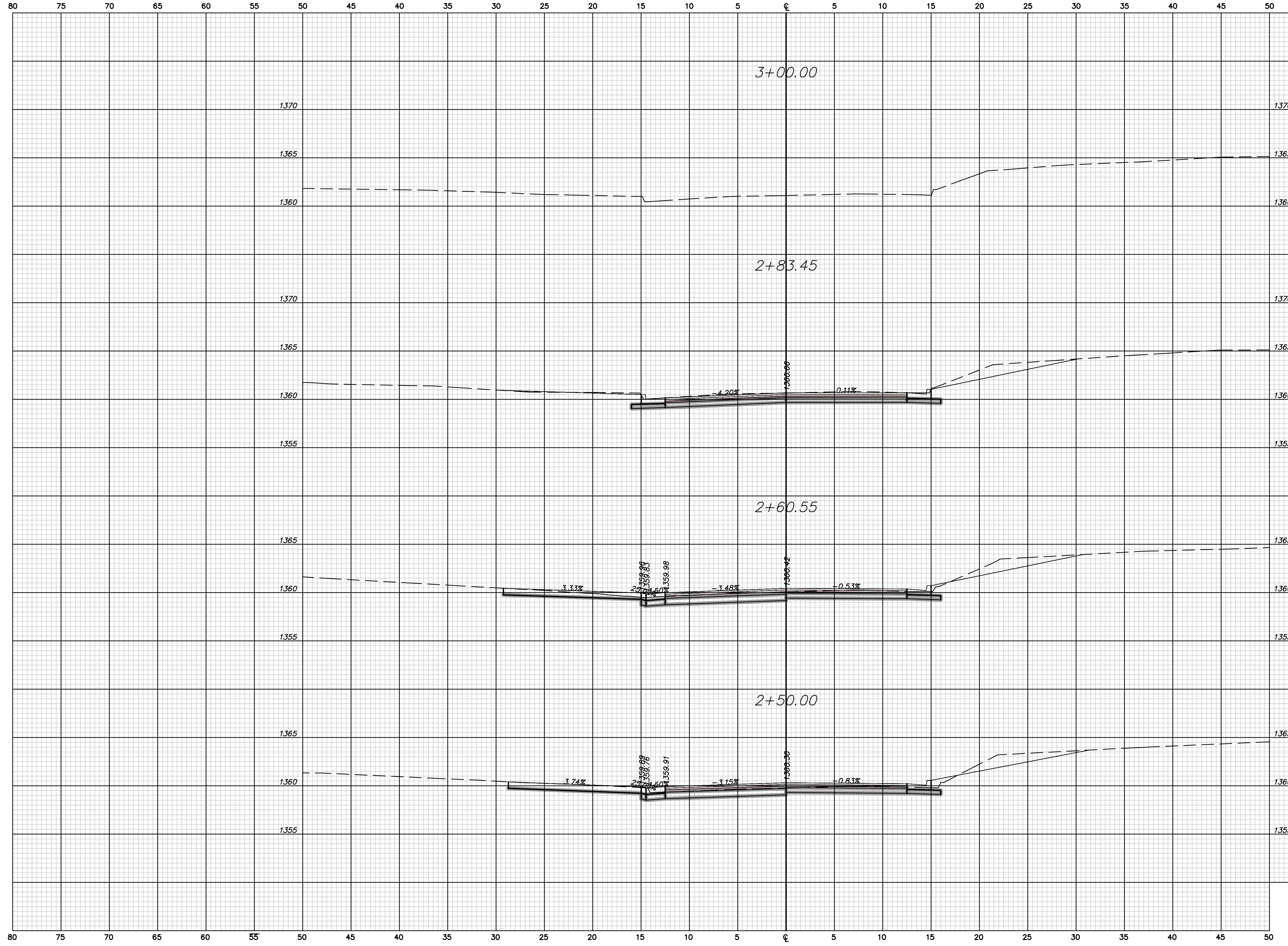
YALE (S. OF 13th ST.) CROSS SECTIONS Sta. 0+50.00 to Sta. 1+00.00
