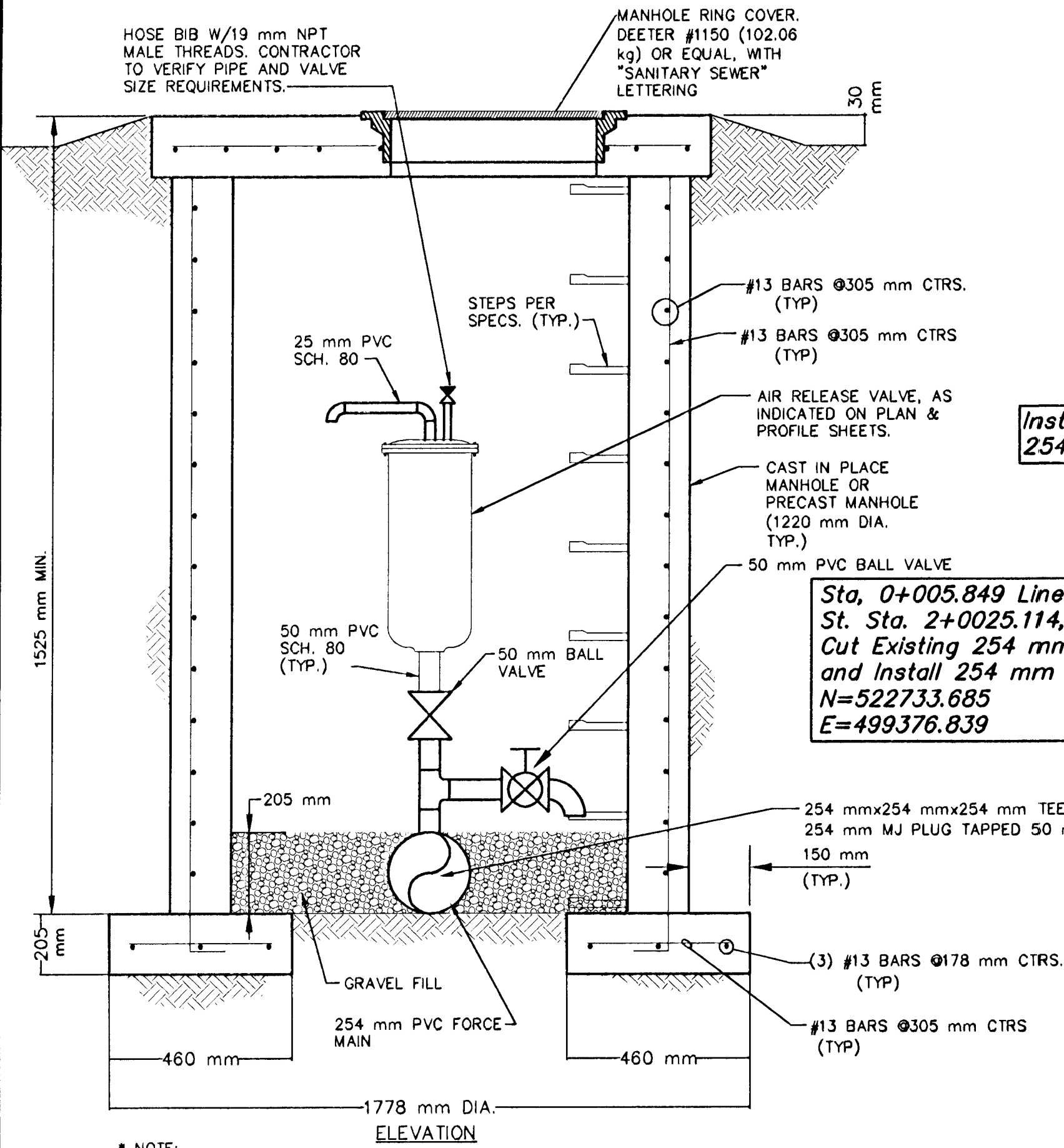
AIR RELEASE MANHOLE N.T.S.
