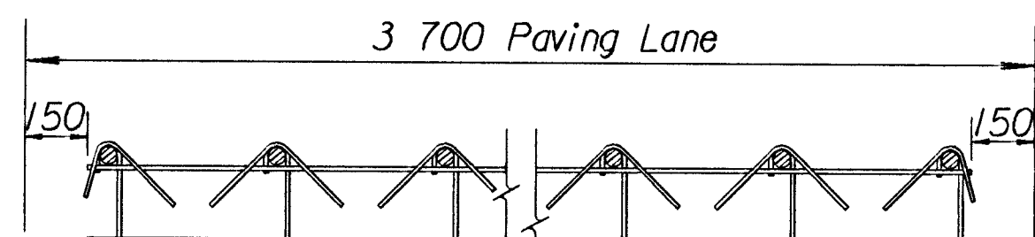
SEC. A-A
