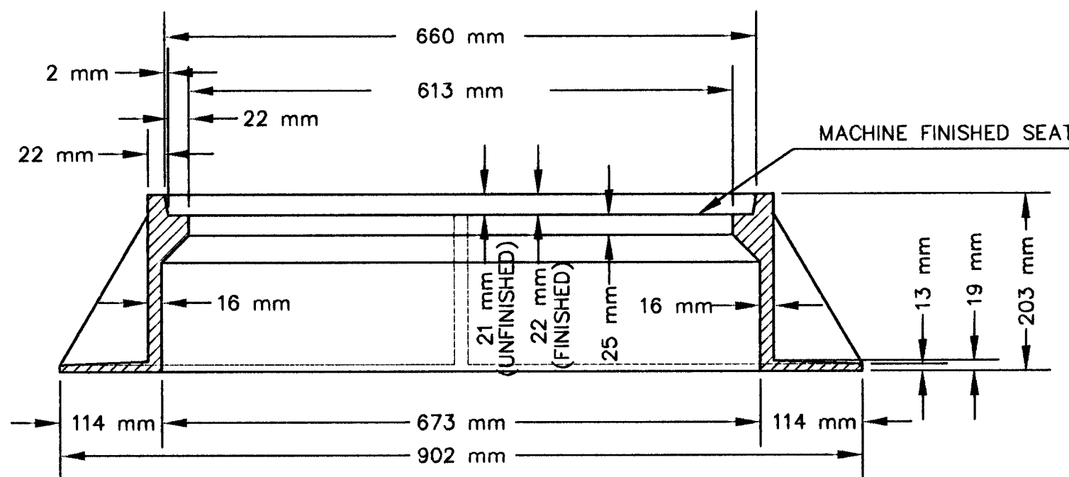
SECTION A-A
