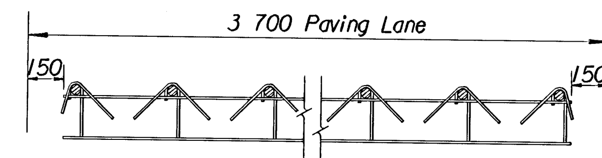
SEC. A-A
