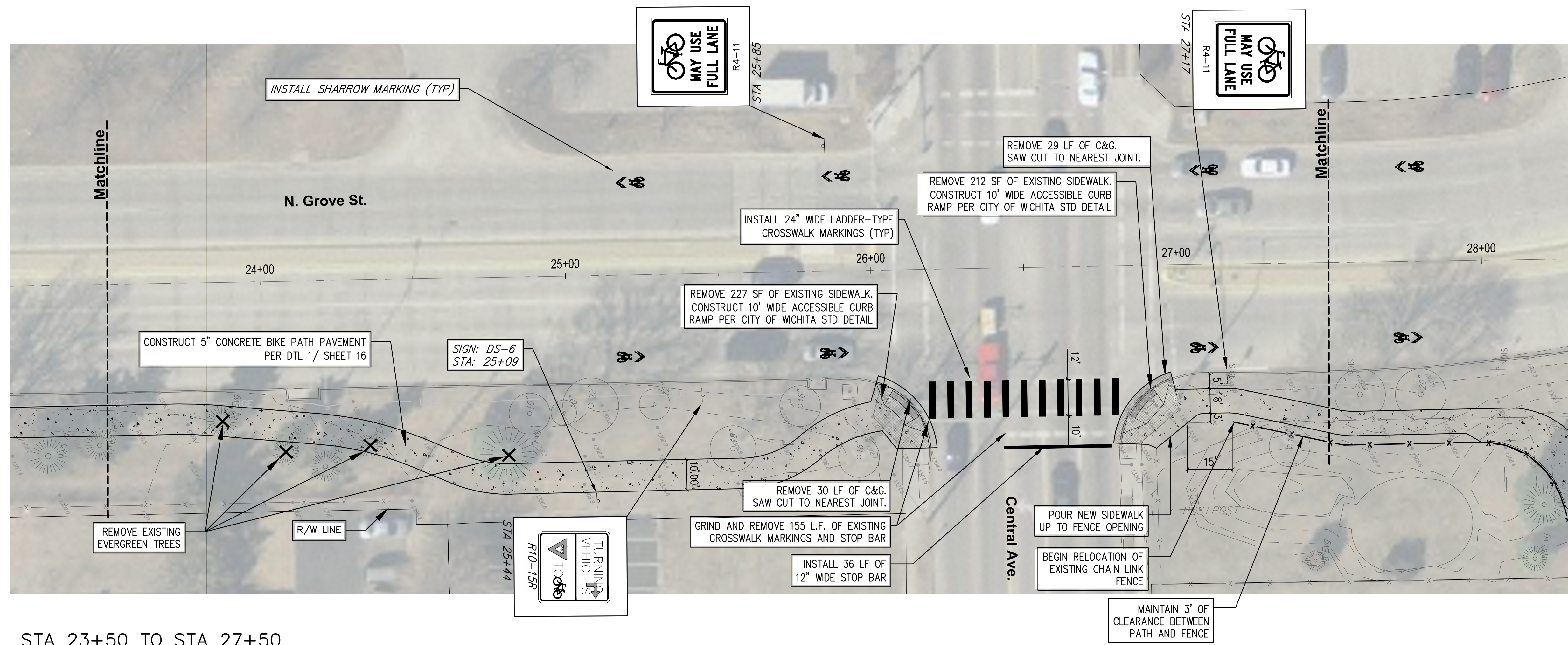
STA 23+50 TO STA 27+50 SCALE 1" = 20' - 0"
