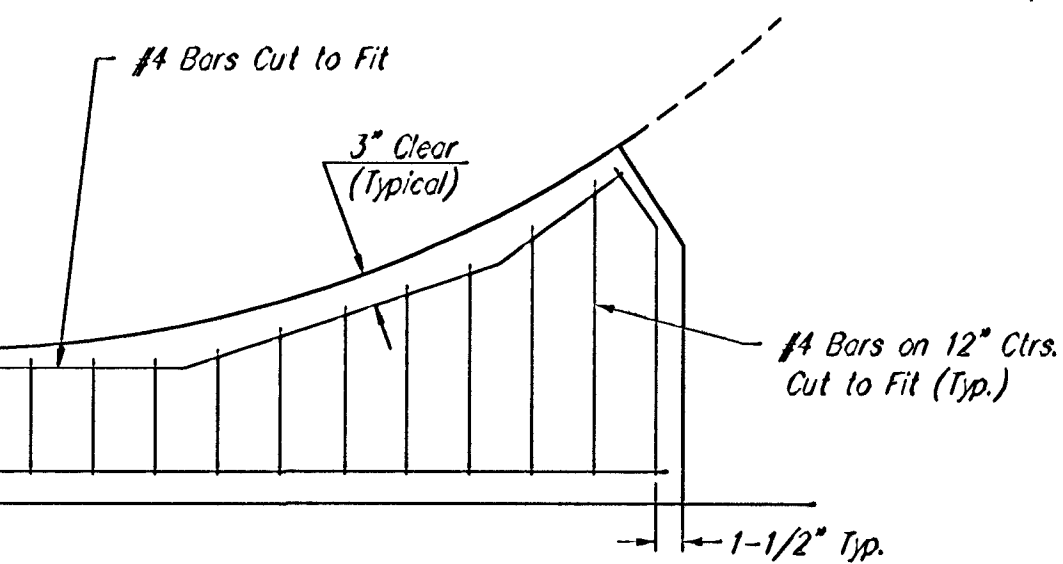
ING REINFORCING DETAIL
