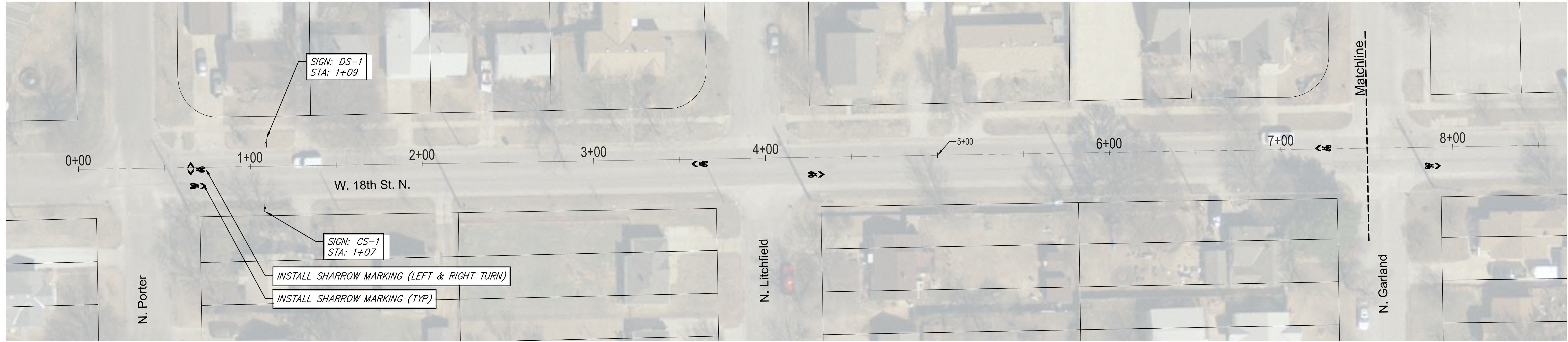
STA 00+00 TO STA 7+50 SCALE 1" = 30' - 0"
