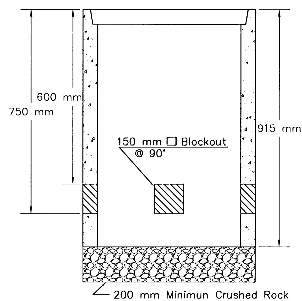
SECTION A-A
