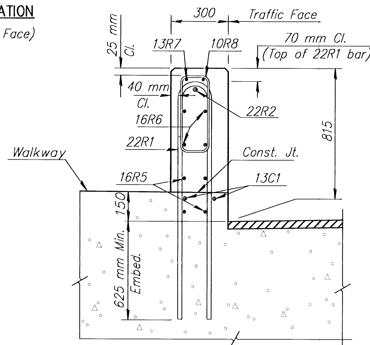
SECTION A-A
