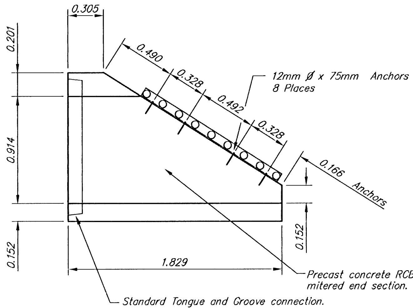
SECTION A-A
