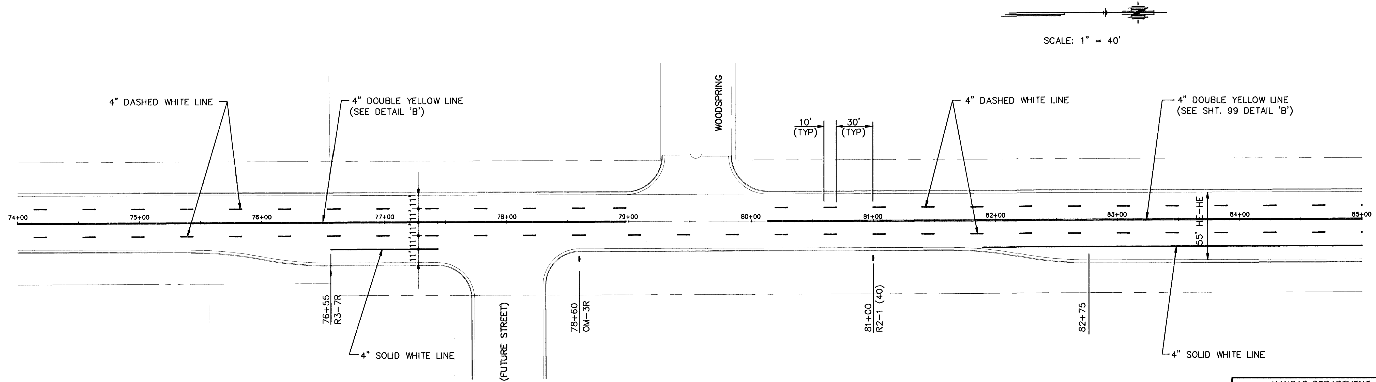
WEBB ROAD - STA 74+00 TO STA 85+00
