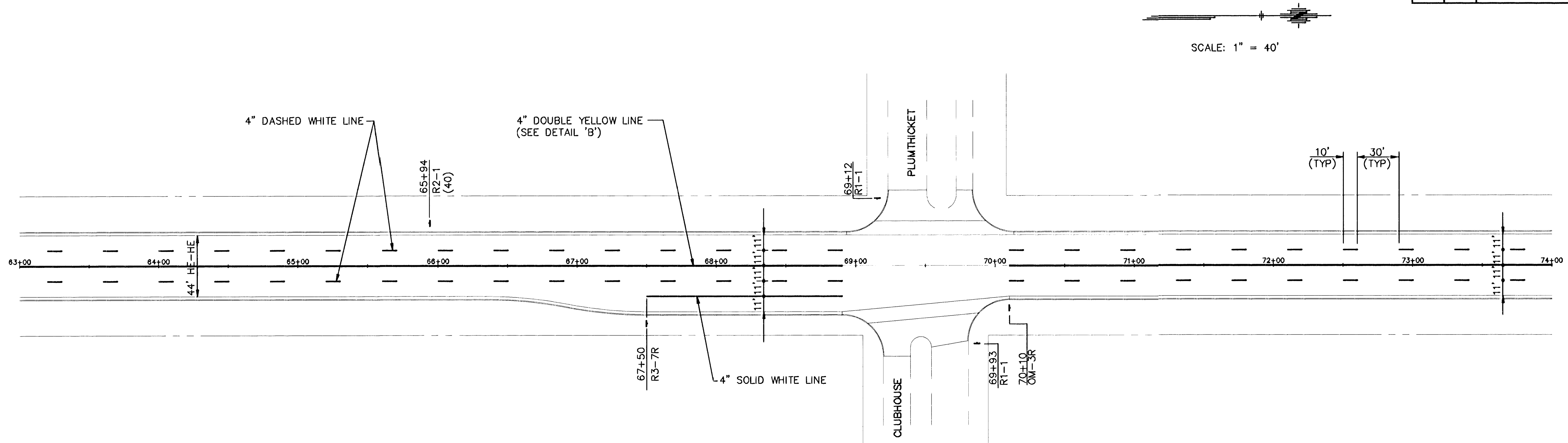
WEBB ROAD - STA 63+00 TO STA 74+00
