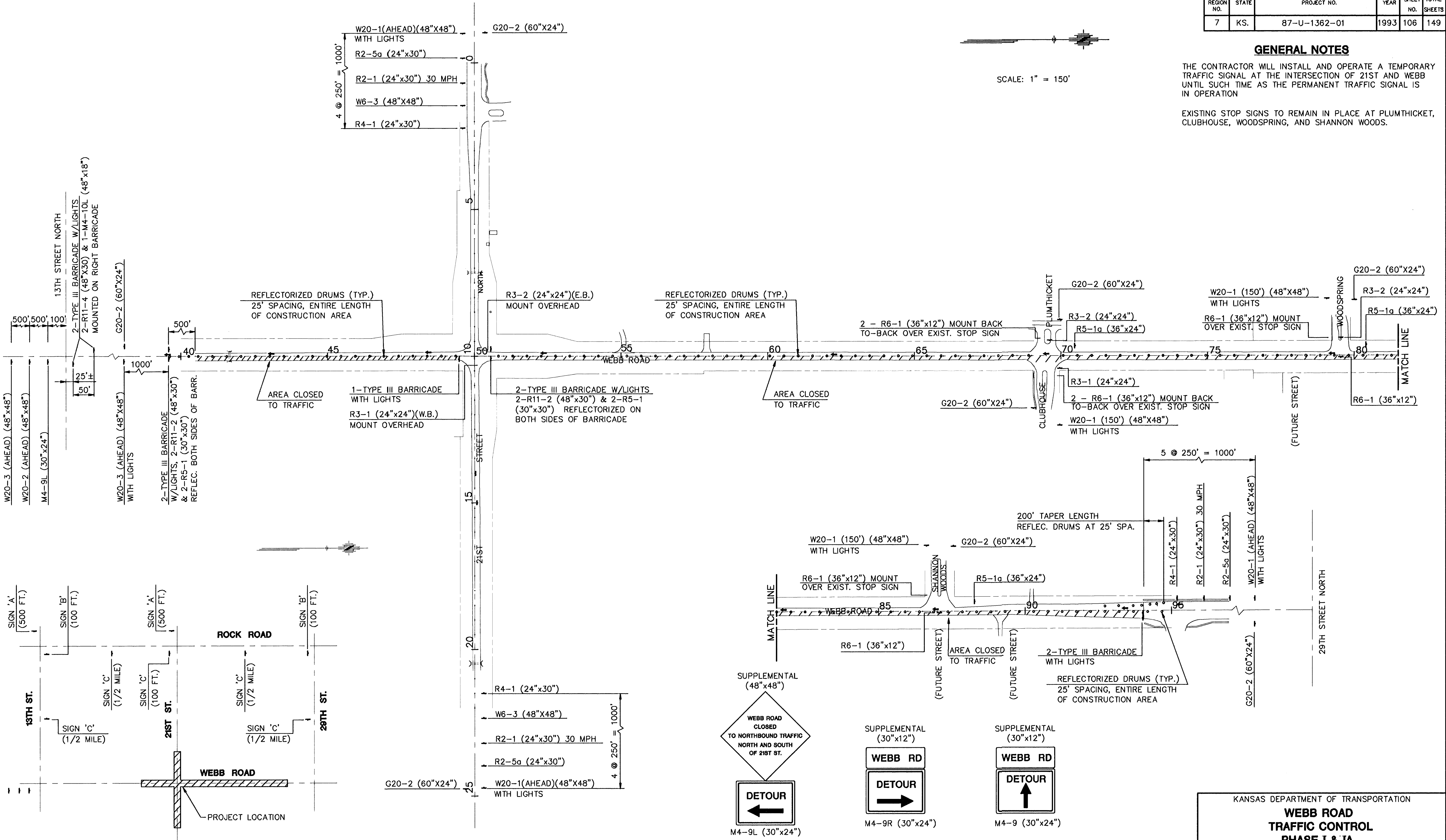
DETOUR PLAN
