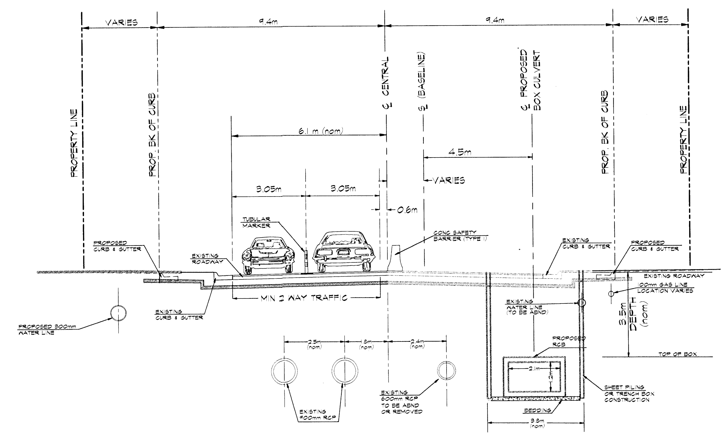
TYP. SECTION
