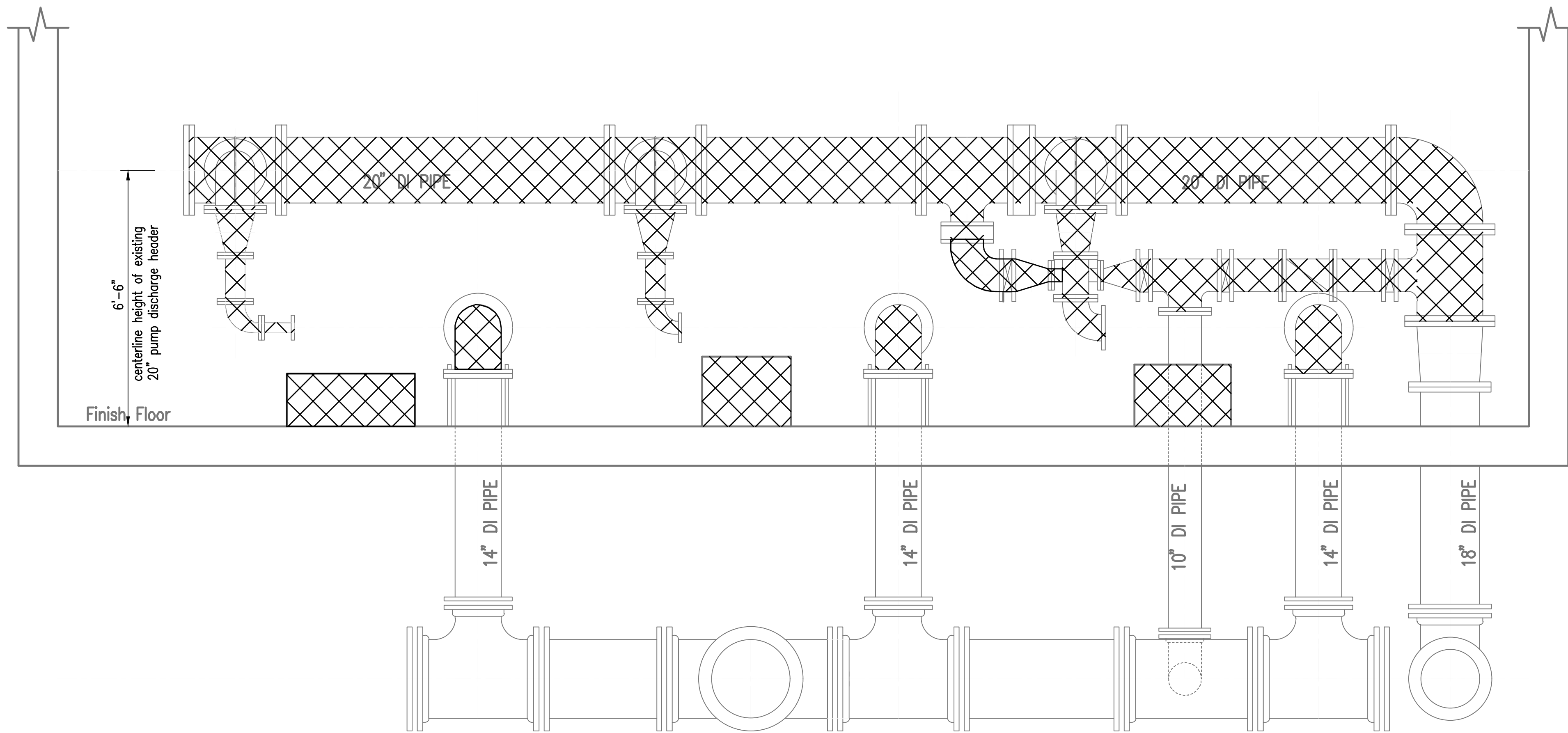
SECTION - MODIFICATION SCALE: 1/2" = 1'-0"
