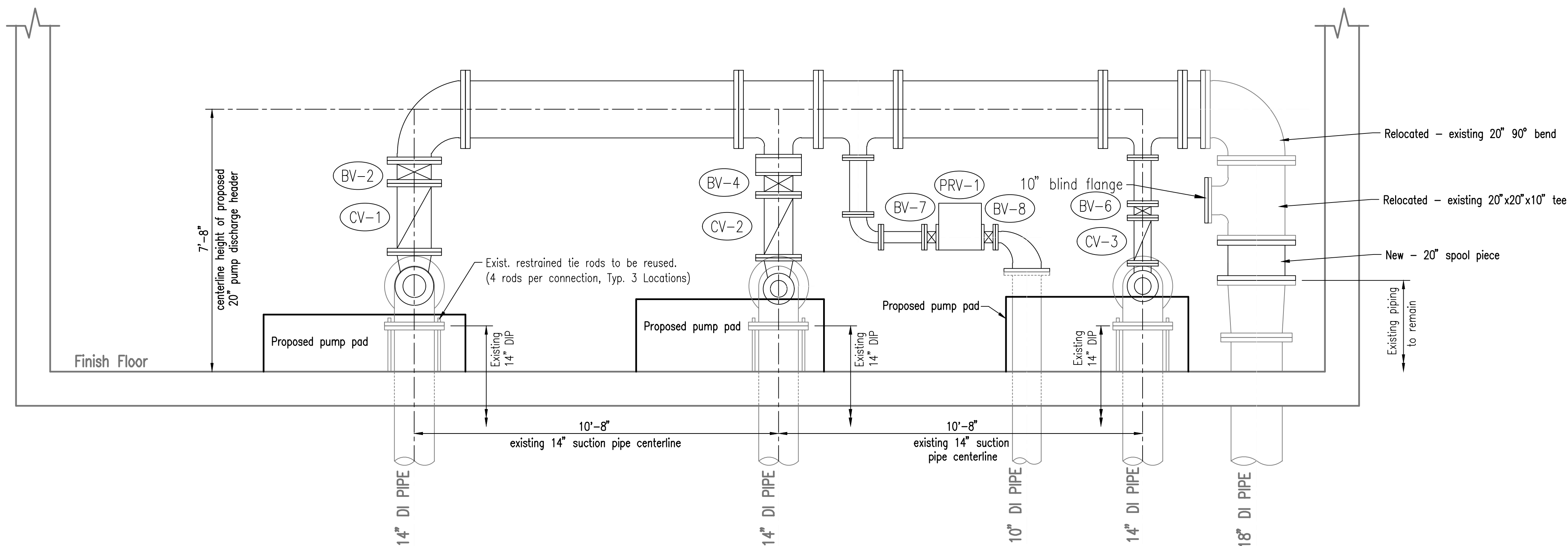
SECTION - MODIFICATION SCALE: 1/2" = 1'-0"
