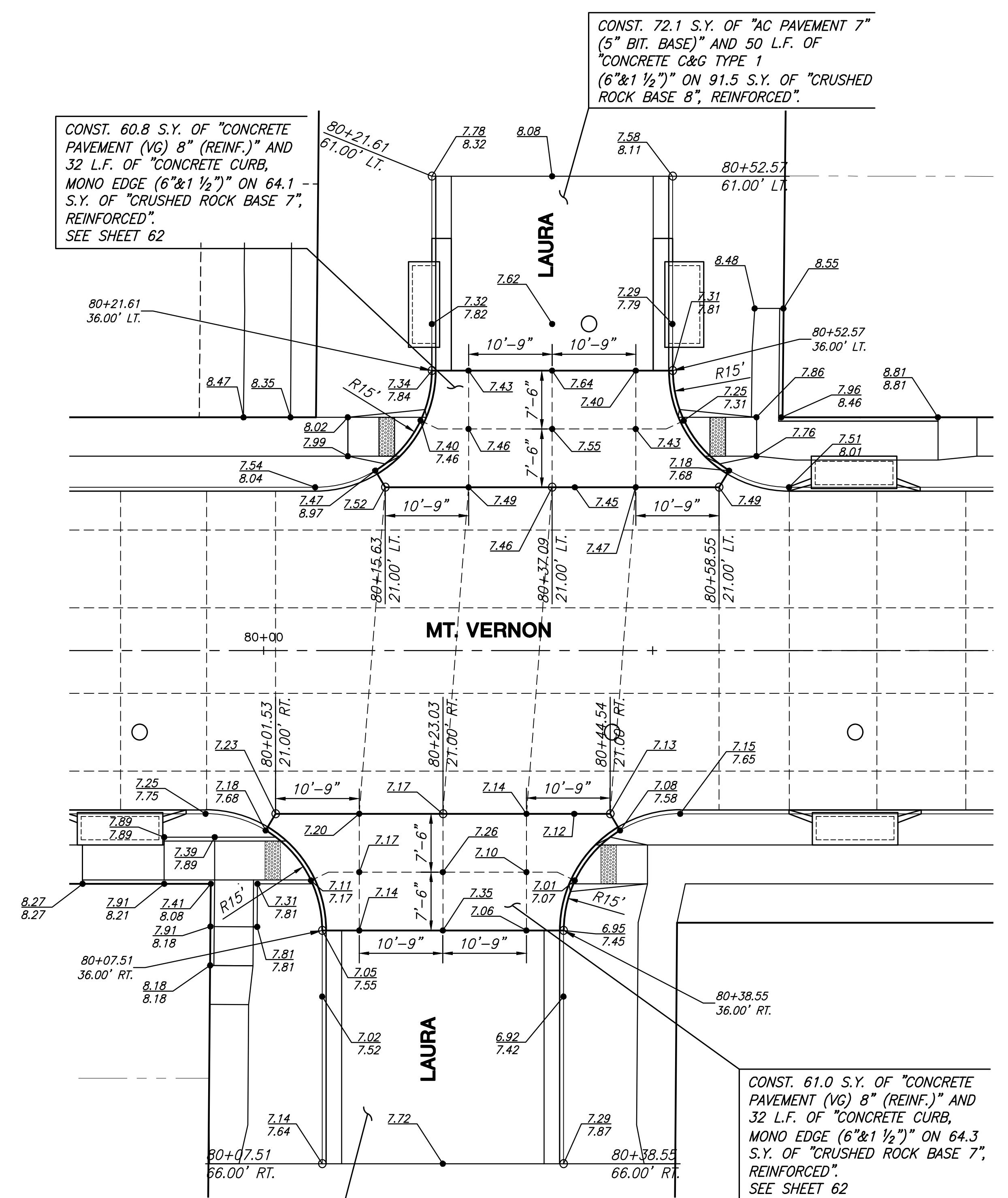
LAURA ST., LT. & RT. SCALE: 1"=10'
