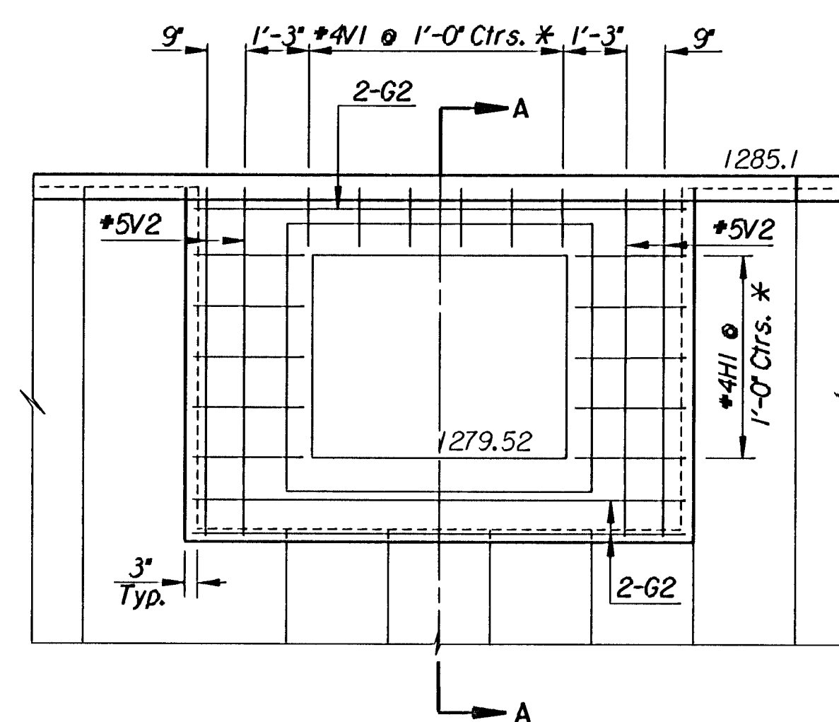
ELEVATION
