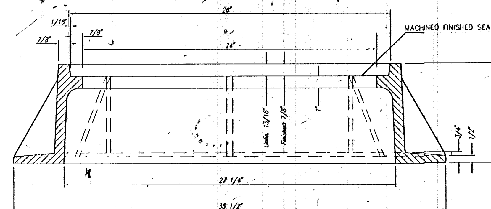
SECTION A-A
