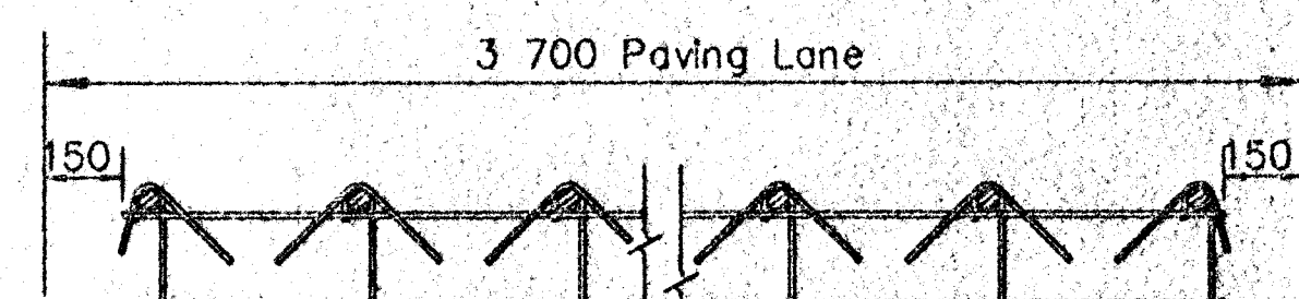
SEC. A-A
