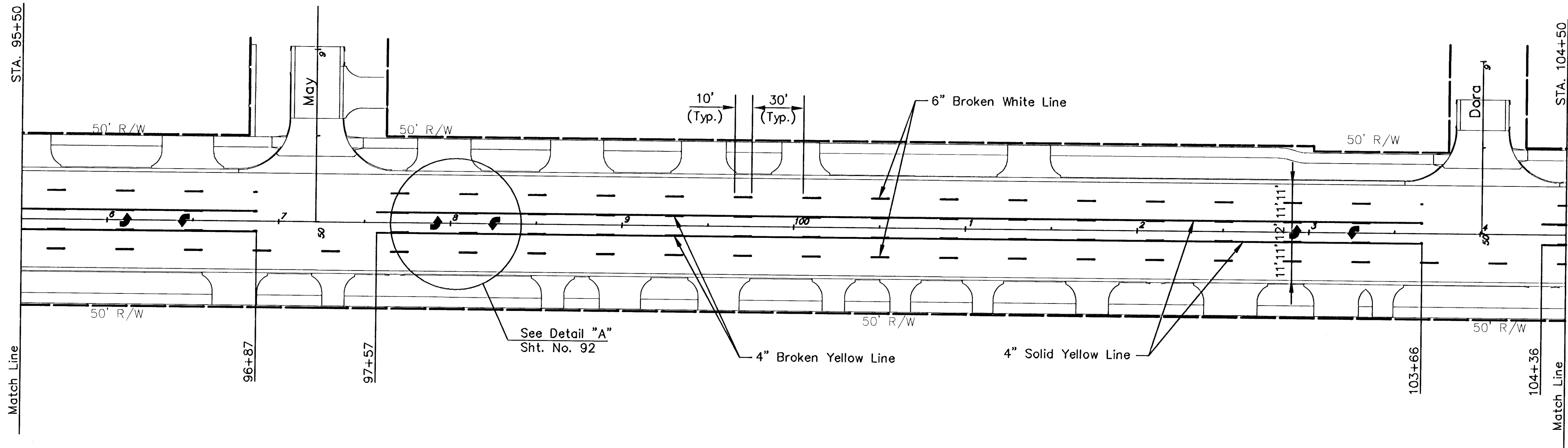
SENECA STREET - STA. 95+50 TO STA. 104+50
