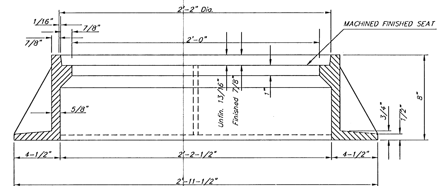
SECTION A-A
