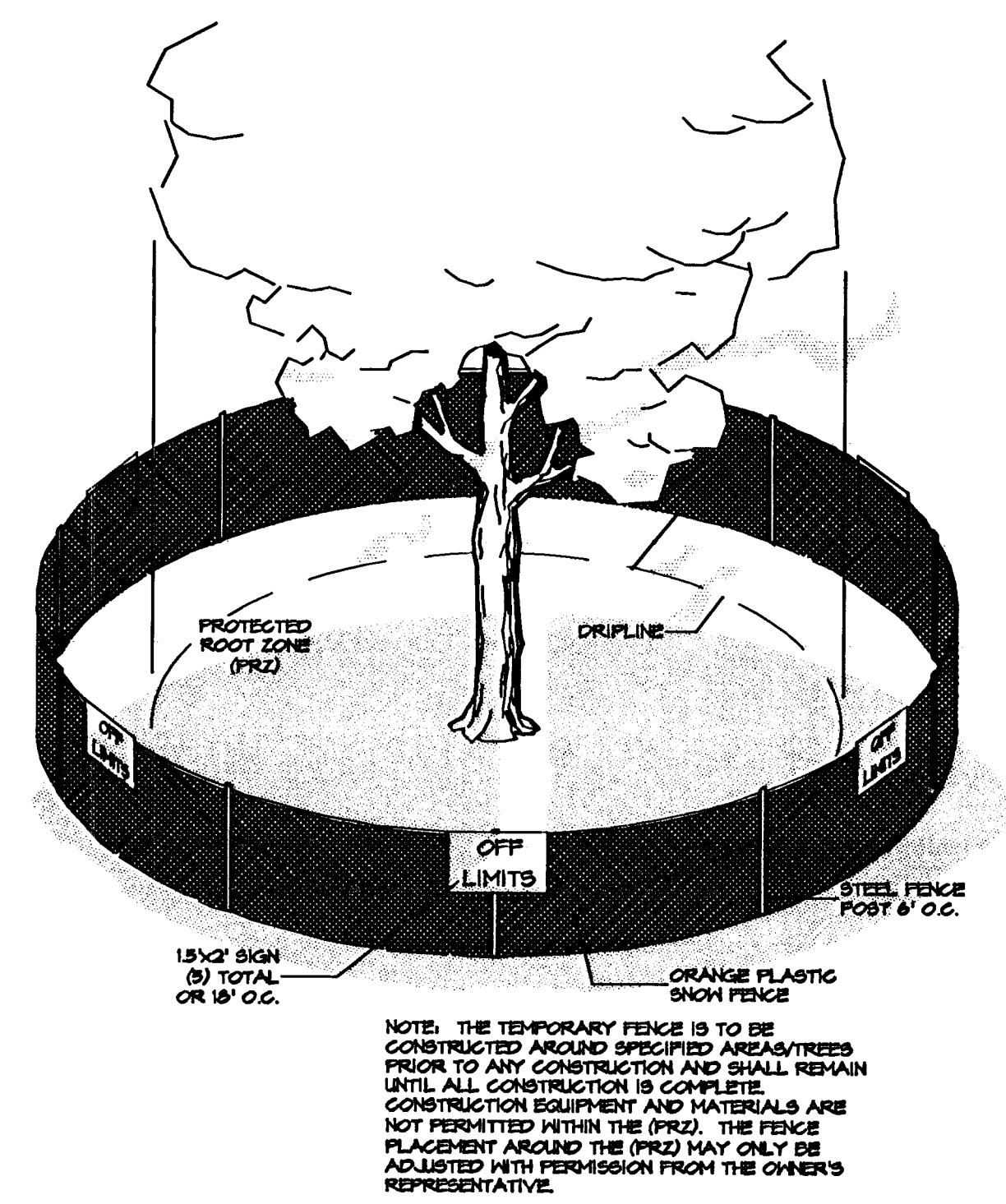
1 TEMPORARY TREE PROTECTION DETAIL SCALE: N.T.S.
