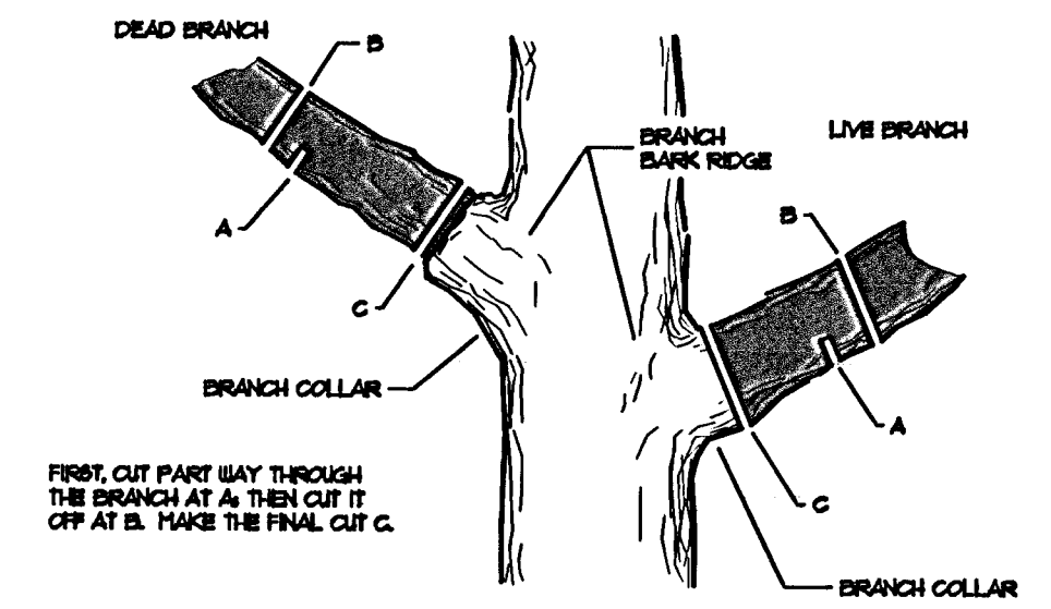
2 TREE TRIMMING DETAIL SCALE: N.T.S.
