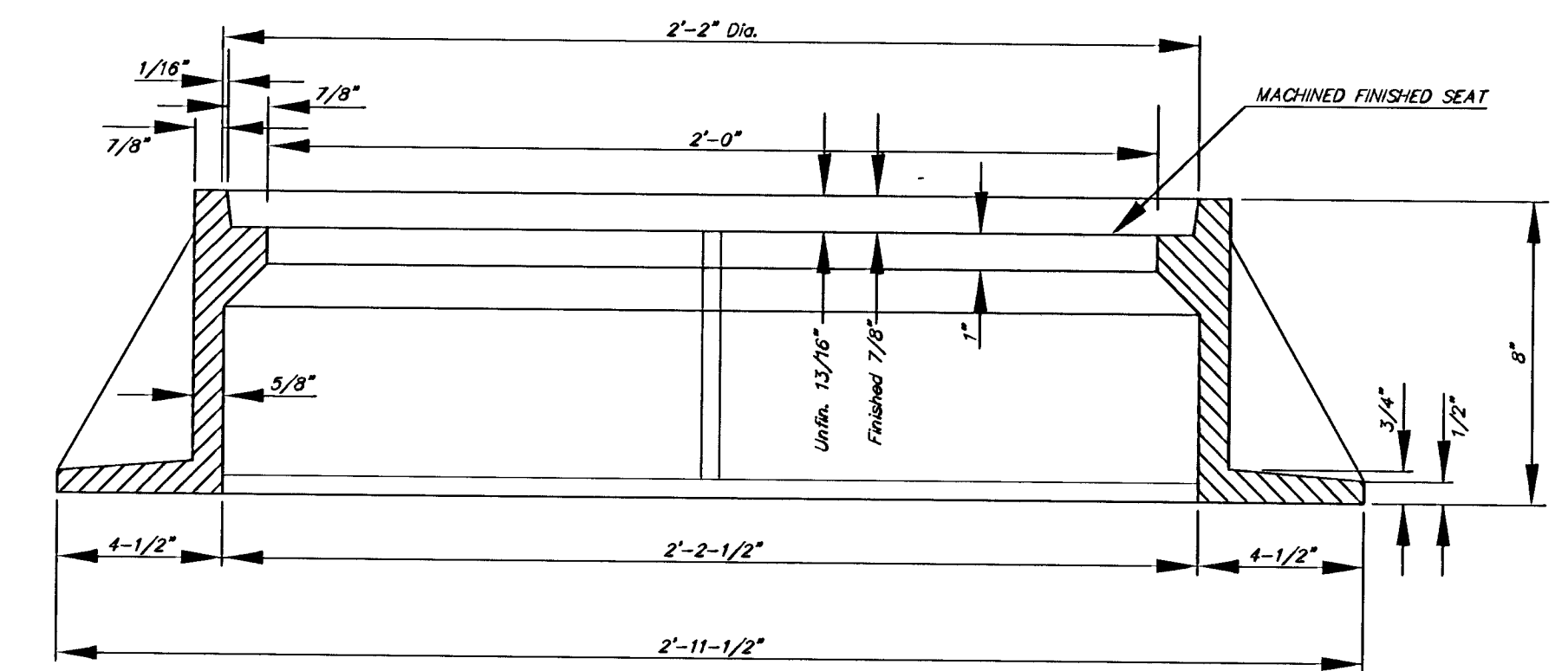
SECTION A-A
